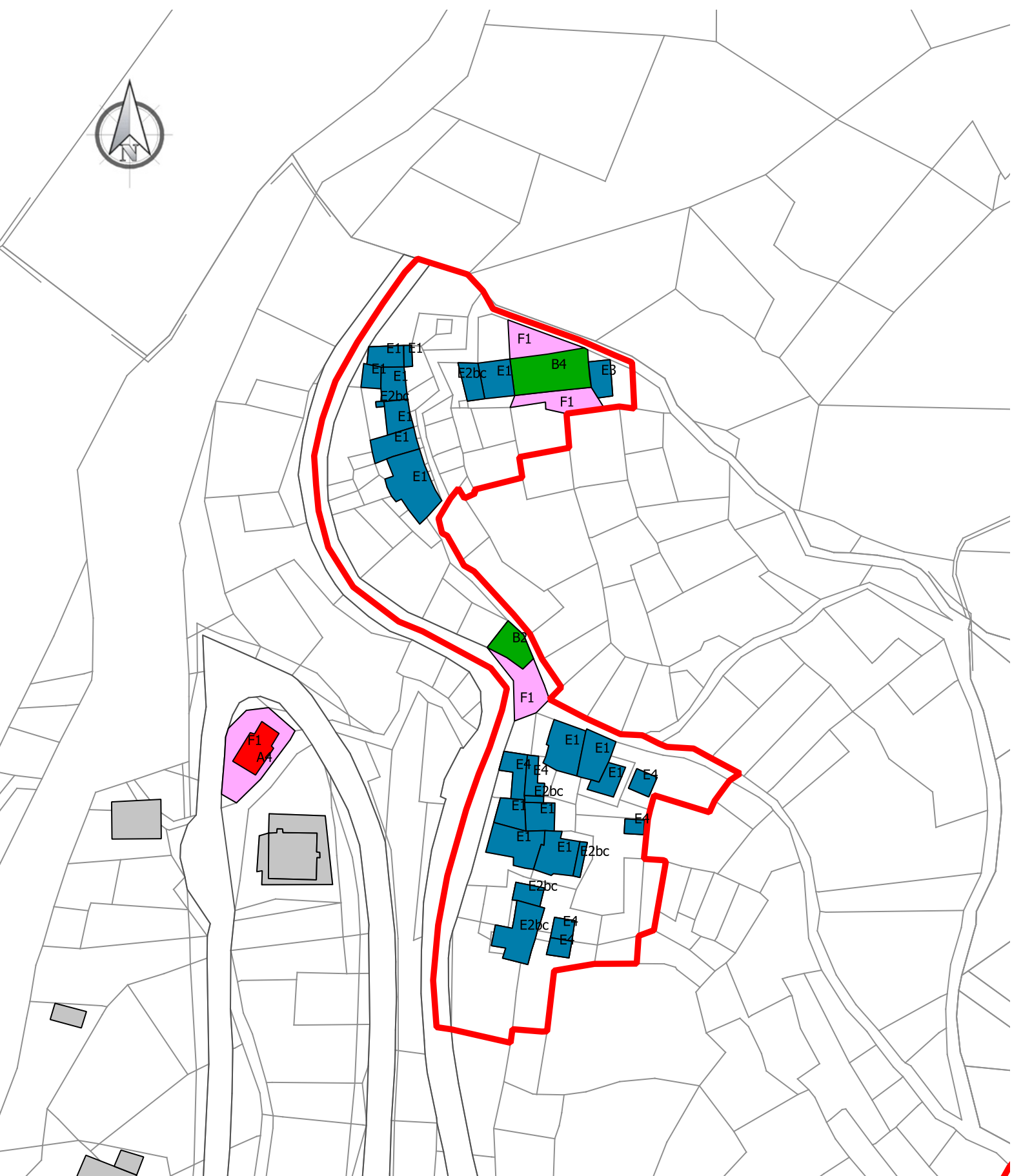
ZONA Ae15 MAISON - NEUVE - TROMEN Scala 1:1000
