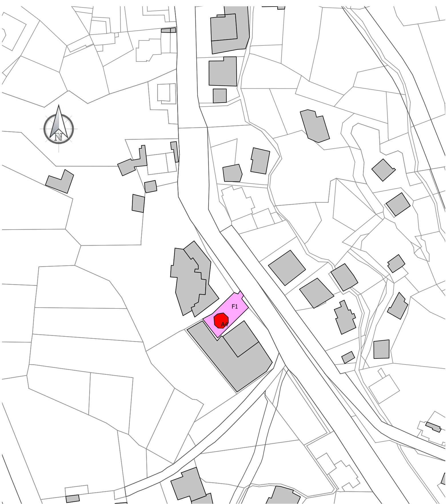
CASE SPARSE CAPPELLA DI PRACOURT Scala 1:1000
